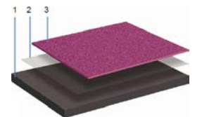
1 Ondergrond 2 Primer (enkel bij beton) 3 Preco Cryl Reibeplastik
