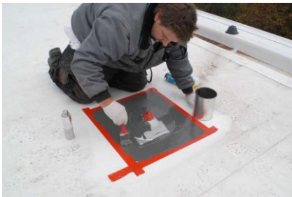
Aanbrengen 2 de laag ProDetail en tape wegnemen
