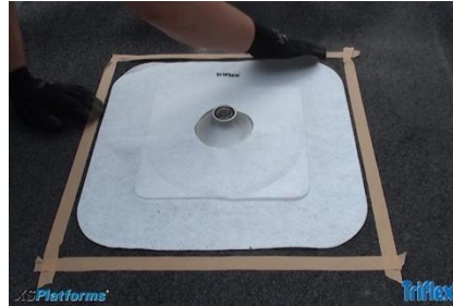
Plaatsen van het voorgevormd vlies en aftapen
